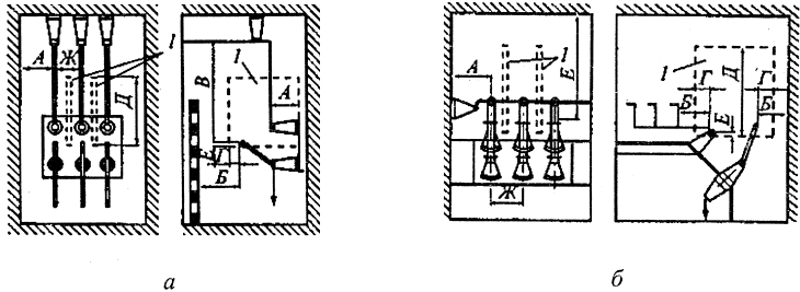
Рис. 4.2.2. Установка разъединителя (отделителя): а — вертикальная; б — наклонная; 1 — изолирующие перегородки
