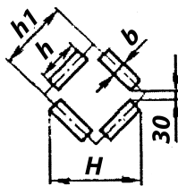
Допустимый длительный ток для четырехполосных шин с расположением полос по сторонам квадрата («полый пакет»)
